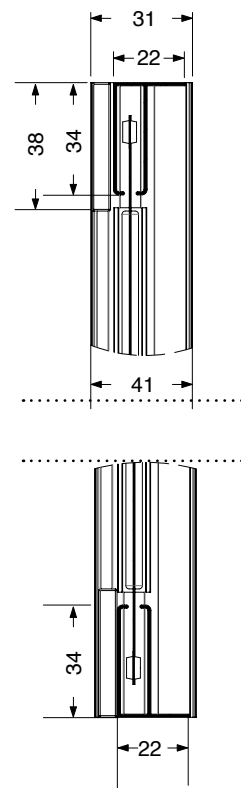
SEZIONE VERTICALE
