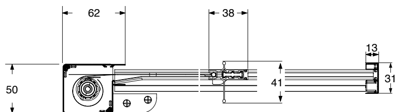
SEZIONE ORIZZONTALE
